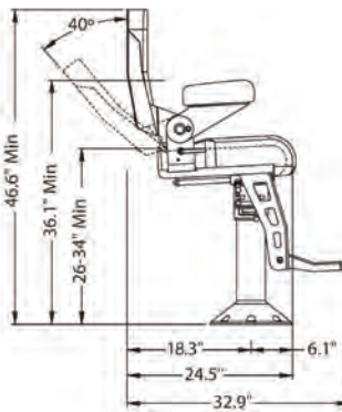
500NX-2X2 & 500N-2X2
